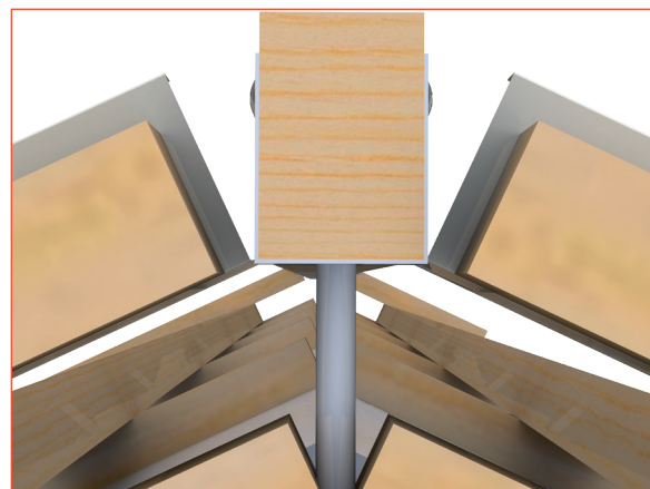
14. Схема размещения подконькового бруса
